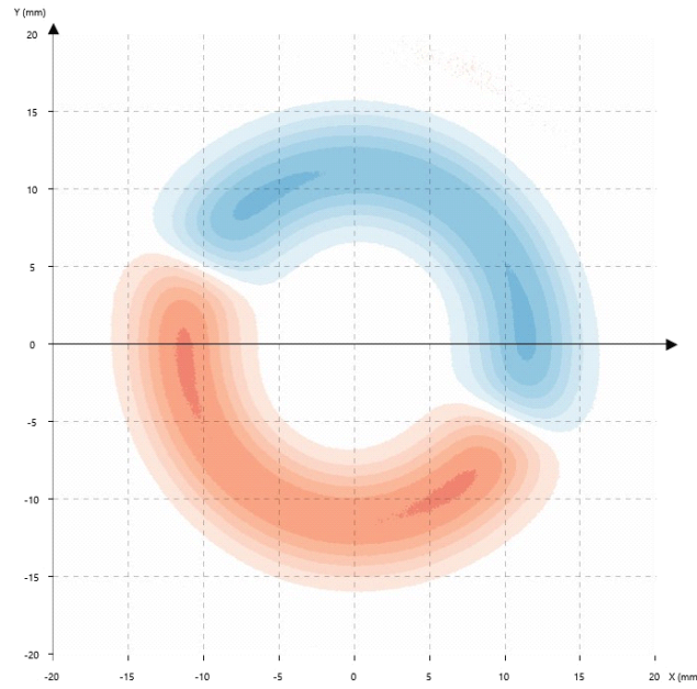
轴向2极圆环
