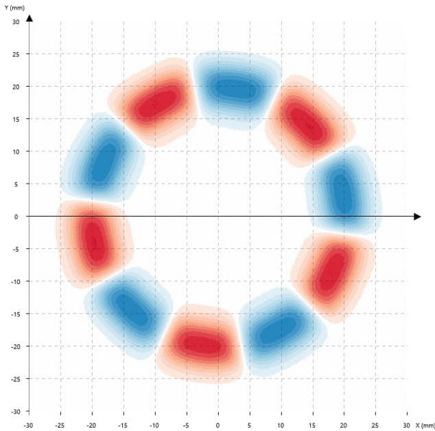
轴向10极圆环
