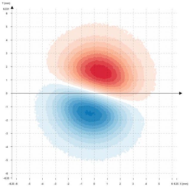
轴向2极圆片
